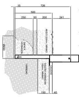
Tipo 1: Zapata pie
