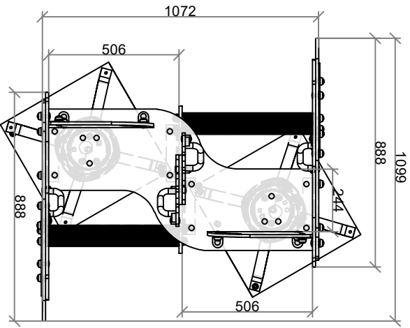
Detalle anclaje suelo pavimento
