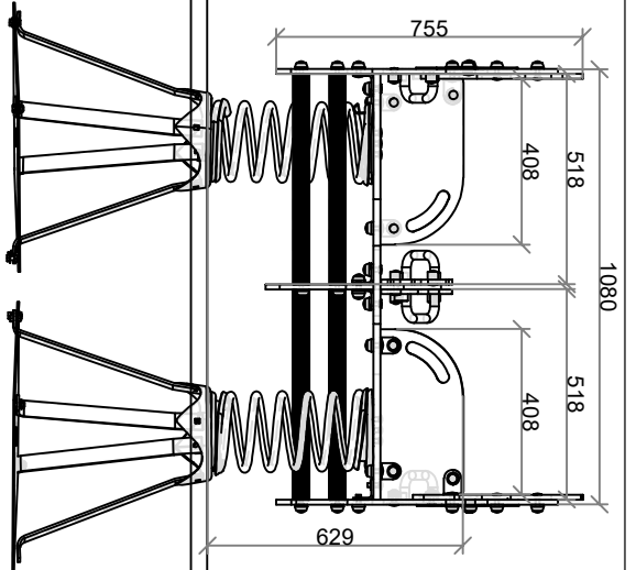
Detalle anclaje suelo pavimento
