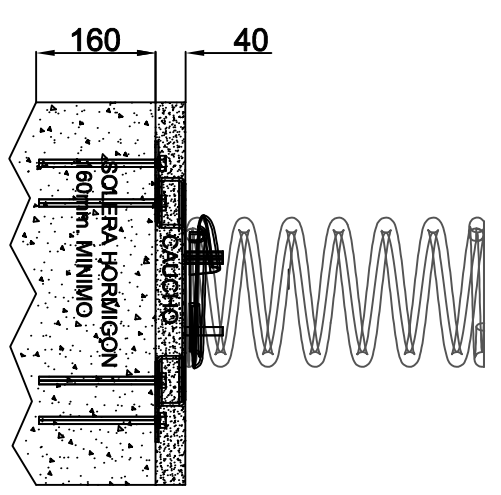
Detalle anclaje suelo pavimento
