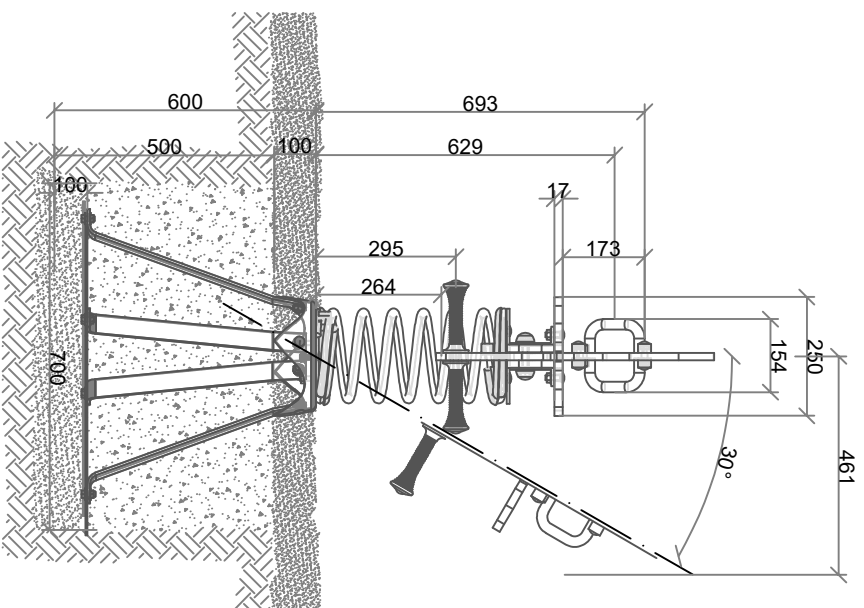
Detalle anclaje suelo pavimento
