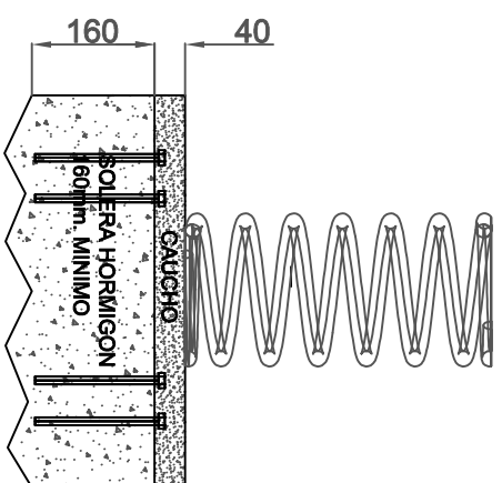
Detalle anclaje suelo pavimento
