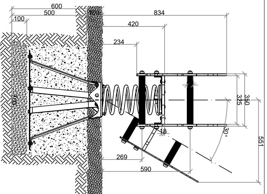
Detalle anclaje suelo pavimento
