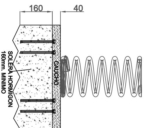
Detalle anclaje suelo pavimento
