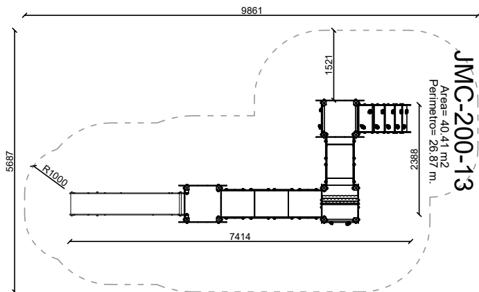
ZAPATA RAMPA CURVADA
