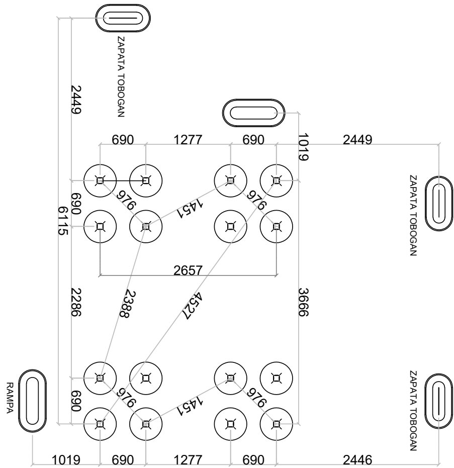
ZAPATA TOBOGAN / RAMPA CURVADA
