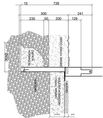
ZAPATA PIE
